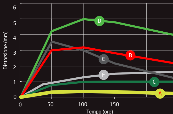
GRAFICO DEL TEST DI STABILITÀ TRADA
