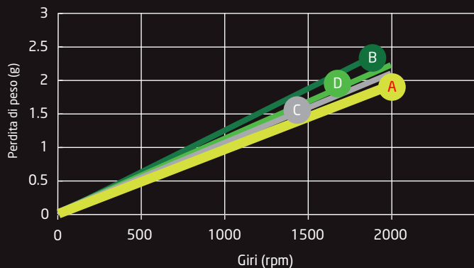
TEST DI ABRASIONE TABER
