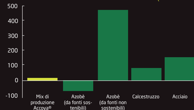
EMISSIONI ANNUE PER OGNI PONTE (KG CO 2 /YR)
