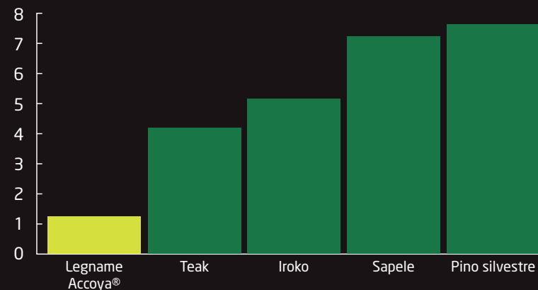
RITIRO TANGENZIALE* (%)
